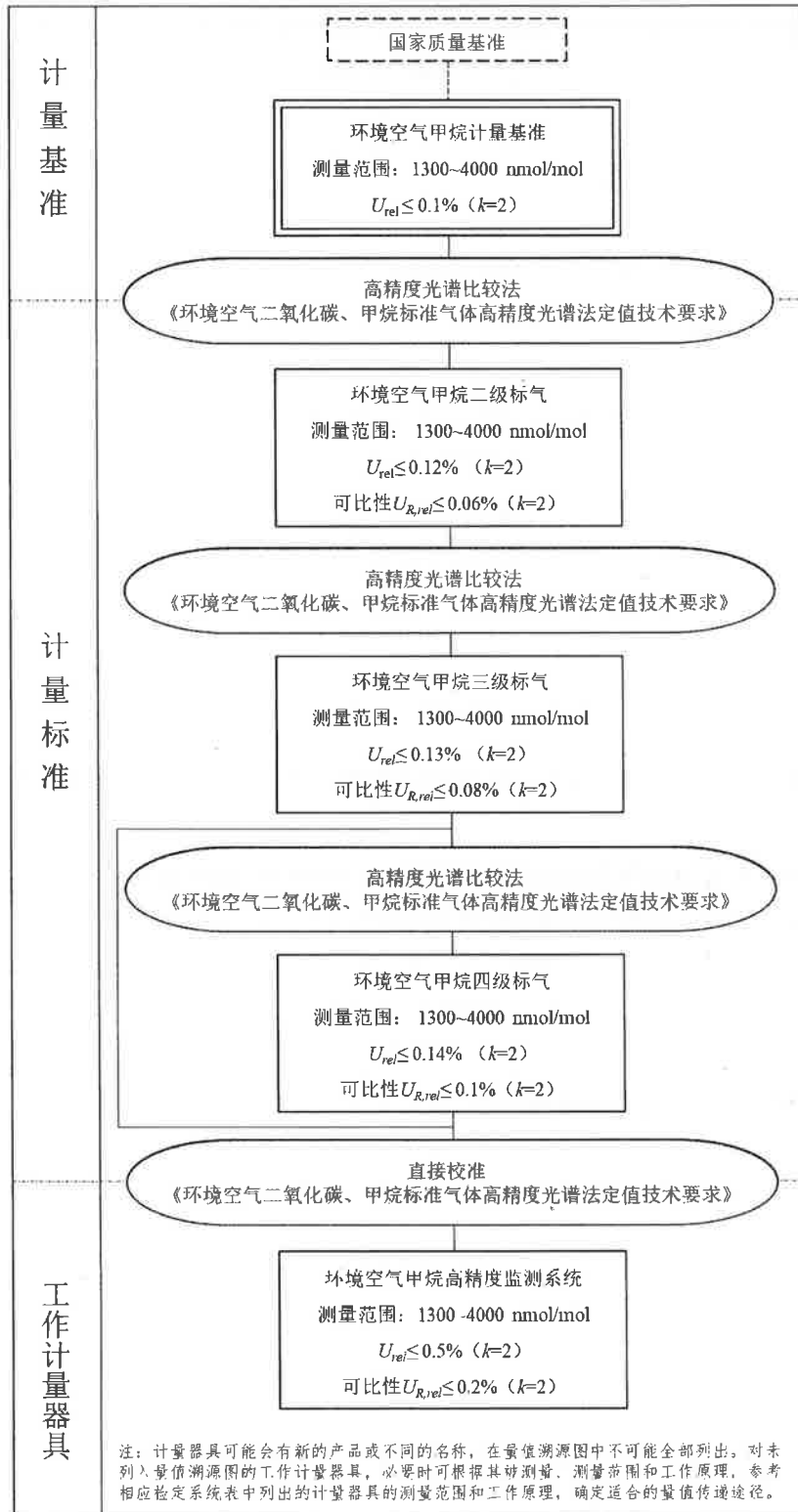
环境空气甲烷高精度监测量值溯源图
